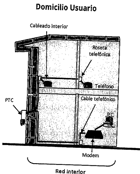
Figura 1. Red Interior de Usuario.
