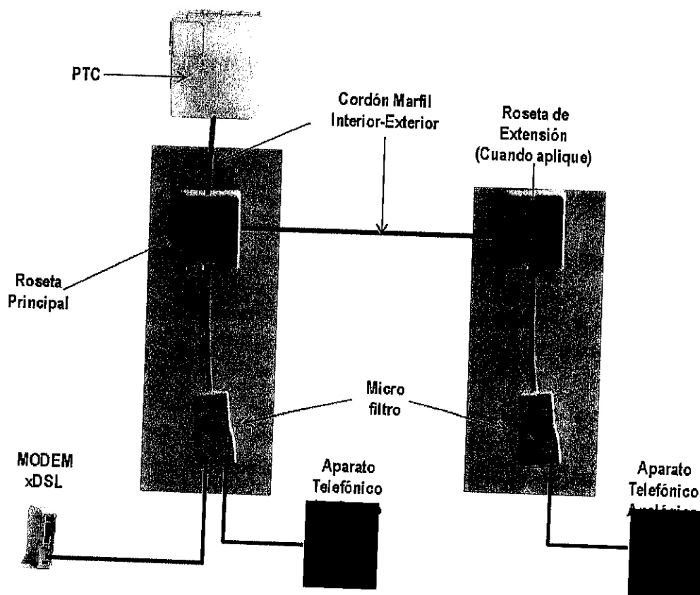
Figura 2. Esquema de la Red interior del Usuario.
