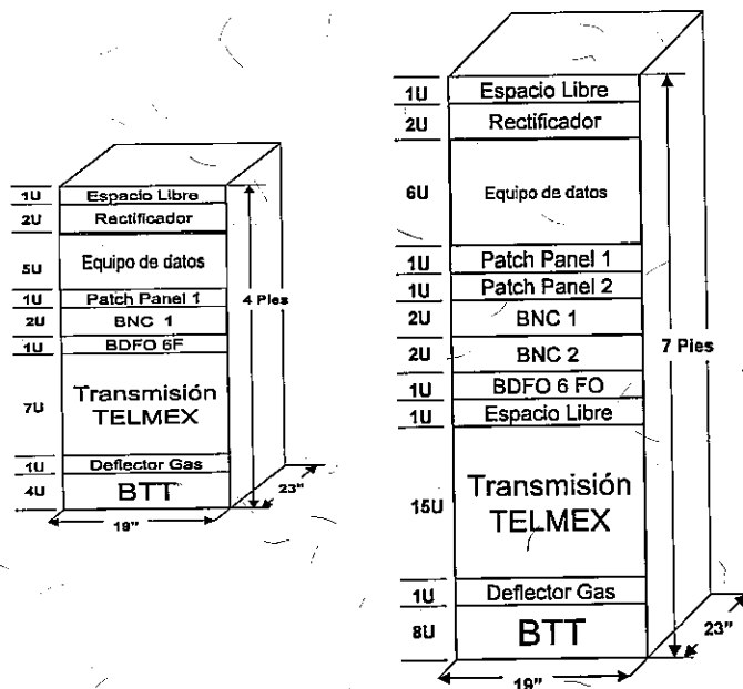
Distribución del gabinete universal Telmex/Telnor
