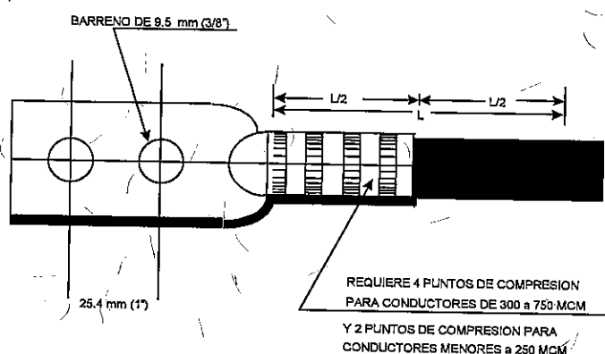
Terminal de Compresión
